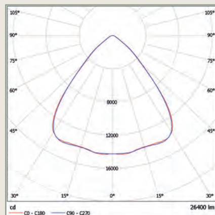
LICHTAUSTRITT ESTD1809090:
