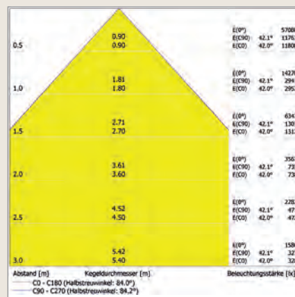
KEGELDIAGRAMM ESTD1809090:
